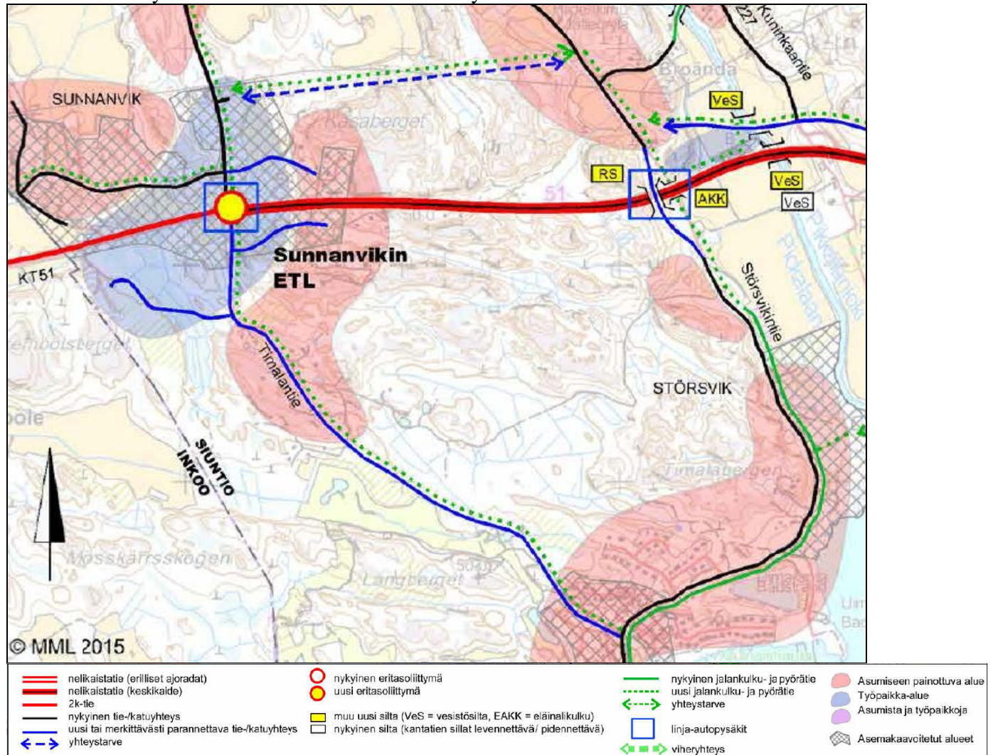
Kantatien 51 parantaminen välillä Kirkkonummi- Inkoon raja, aluevaraussuunnitelma, A-Insinöörit 2017
